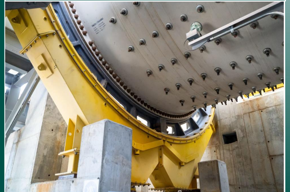
Molino SAG.
